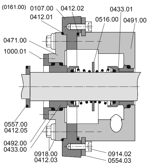
Рис. 25: Двойное механическое уплотнение, параллельное, седло B2.
