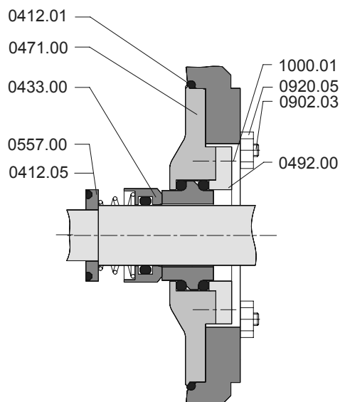
Рис. 12: Оди́нарное механическое уплотнение, седло В3.
