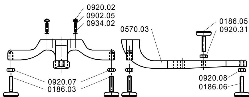
Рис. 40: Комбинированная подставка BG2
