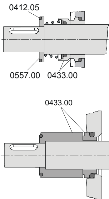
Рис. 10: Одинарное механическое уплотнение
