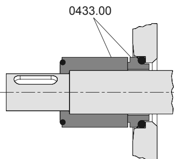
Рис. 30: Стерильное механическое уплотнение
