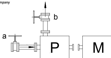
Рис. 8: Клапанный блок
