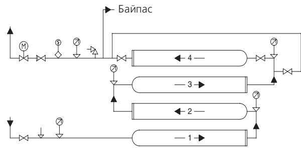
Рис. 8 Блок из четырех последовательно включенных бустерных модулей с байпасной линией, размещенных друг над другом.
