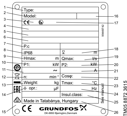
Рис. 1 Фирменная табличка
