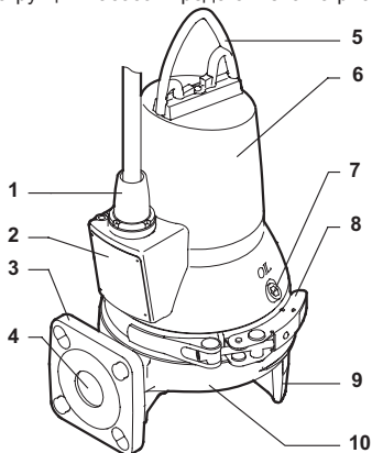
Рис. 1 Насос SEG
