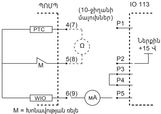
Նկար 17 SE1 և SEV պոմպեր PTC տվիչով
