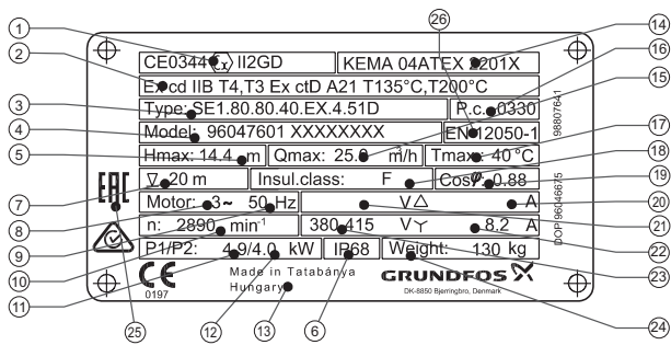
Նկար 2 Ֆիրմային վահանակ
