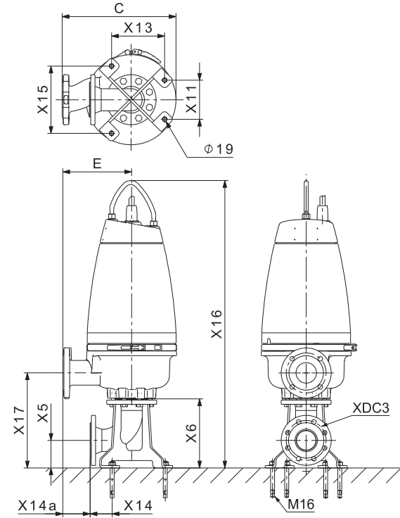
Рис. 41 Сухая установка насоса SEV в вертикальном положении
