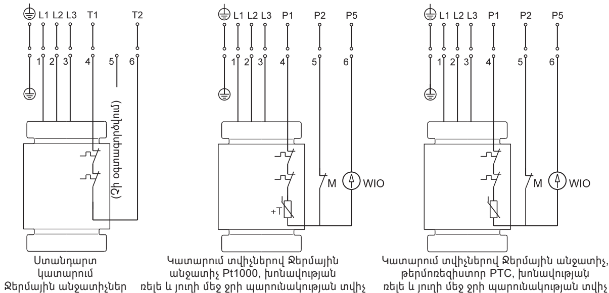
Նկար 9 Էլեկտրական միացումների սխեմաները 7 ջիղանի մալուխի համար, անմիջական գործարկում
