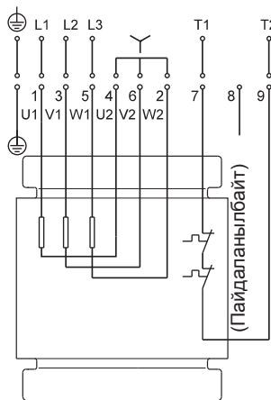
Стандарттык аткарылышы Термөөчүргүч
