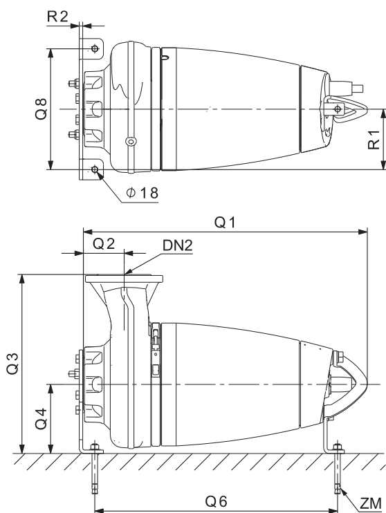
Рис. 36 SE1 Сухая горизонтальная установка
