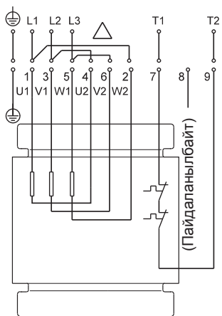
Стандарттык аткарылышы Термөөчүргүч
