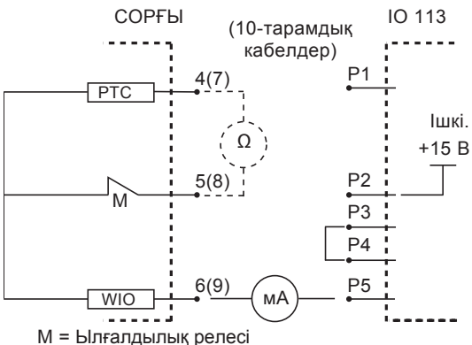
17-сур. PTC датчигімен SE1, SEV сорғылары
