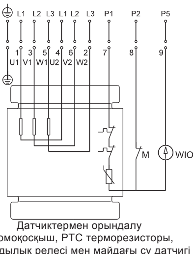
10-сур. 10-тарамдық кабель үшін электр қосылыстардың схемалары, «жұлдызша-ұшбұрыш» (Y/D) қосылысы
