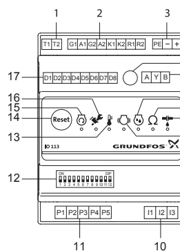
Рис. 15 Модуль IO 113
