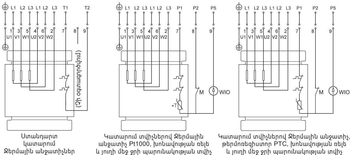
Նկար 10 Էլեկտրական միացումների սխեմաները 10 ջիղանի մալուխի համար, միացում ,աստղ և եռանկյուն (Y/D)
