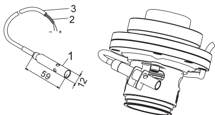
14-сүр. WIO билдиргичи
