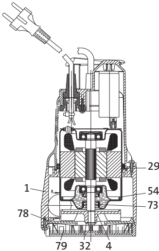
Рис. 1 Разрез насоса KPC
