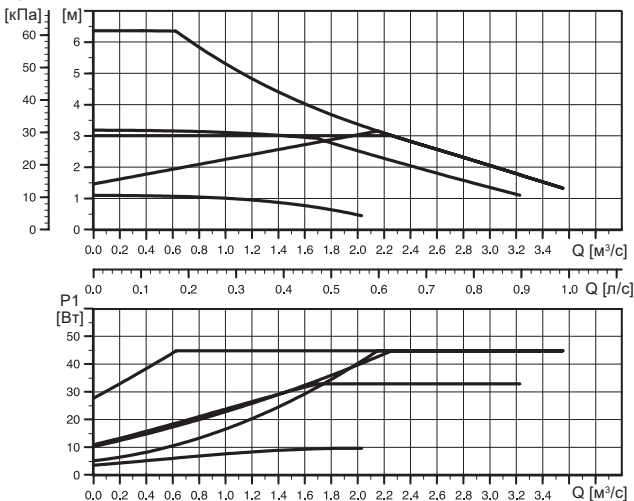
18-сур. ALPHA1 L сериясындағы сорғылардың шығынды-арынды сипаттамасы
