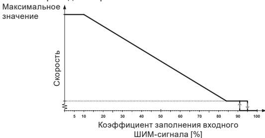
Рис. 14 Профиль управляющего ШИМ-сигнала в ALPHA1 L
