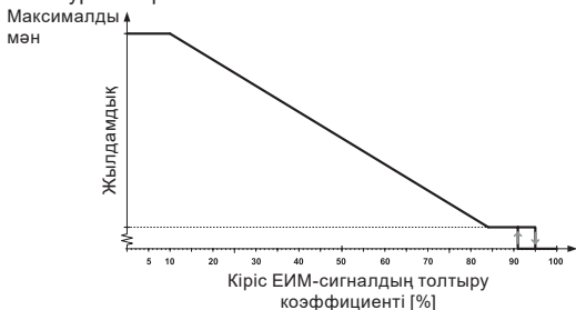
14-сур. ALPHA1 L басқарушы ЕИМ-сигналдың бейіні
