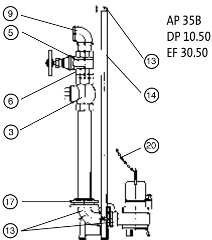
Комплектация с резьбовыми соединениями
