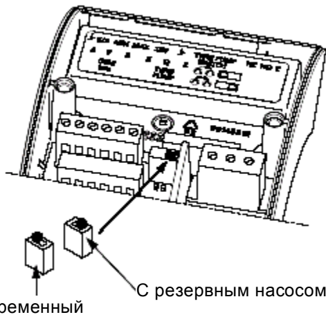
Рис. 9 Коммутационная переключатель
