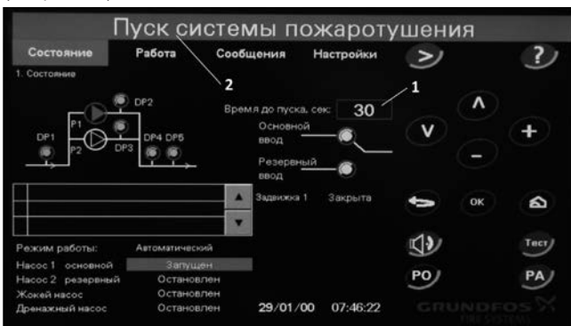
Рис. 14 Меню «Состояние» при поступлении сигнала на запуск
