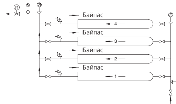
7-сур. Төрт параллель қосылған, бір-біріне орналастырылған бустерлік модульден тұратын блок
