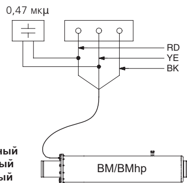
Рис.11 Подсоединение конденсатора
