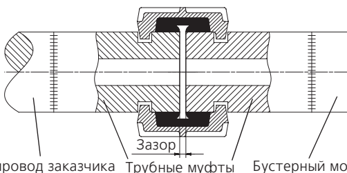
Рис. 10 Трубная муфта типа Victaulic/PJE
