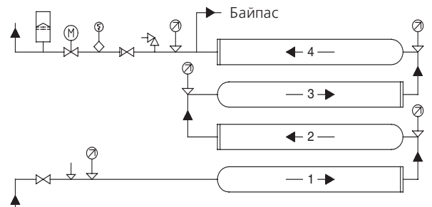
6-сур. Төрт жүйелі түрде қосылған, бір-біріне орналастырылған бустерлік модульден тұратын блок
