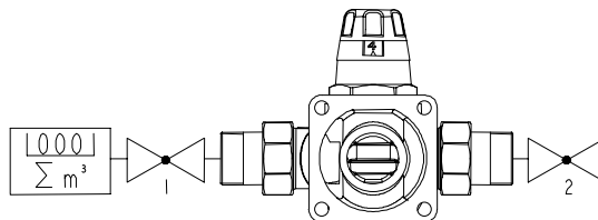
Рис. 1: Горизонтальный монтаж
