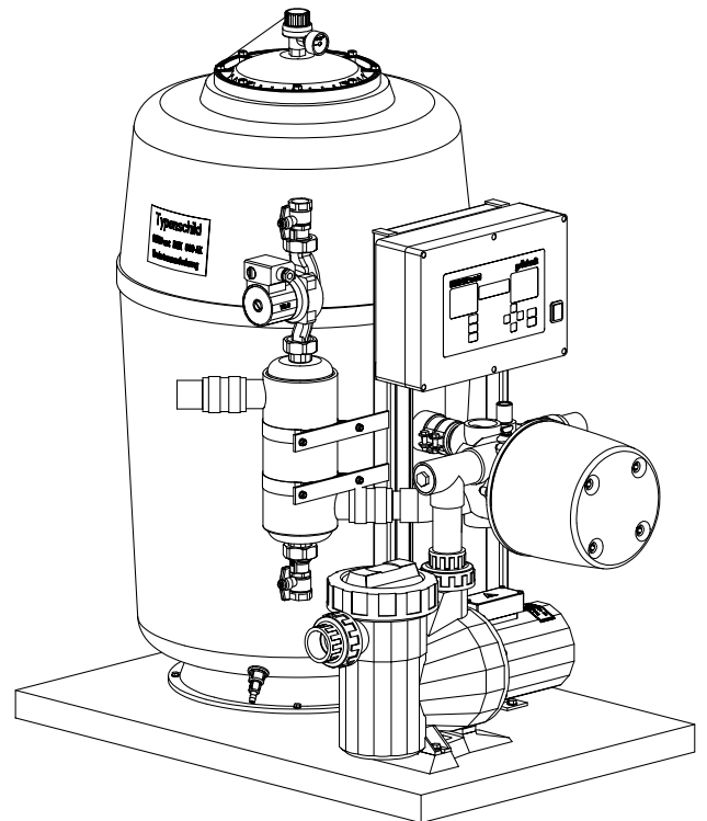
Фильтровальные установки GENO-mat® BWK 500 AK / BWK 600 AK
