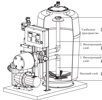
Рис. 7с: BWK 600 AK с кварцевым песком и гидроантрацитом "N"
