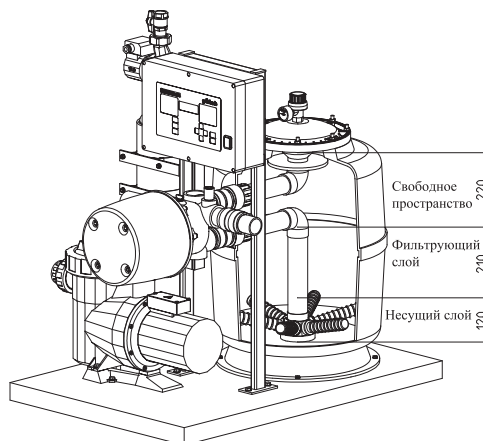
Рис. 7а: BWK 500 AK с кварцевым песком
