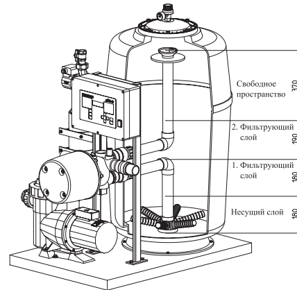
Рис. 7b: BWK 600 AK с кварцевым песком
