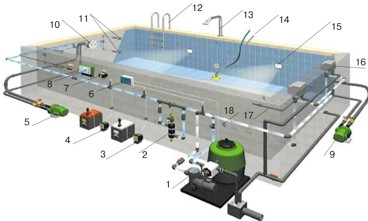
Рис. 3: Пример монтажа в бассейне со скиммерами
