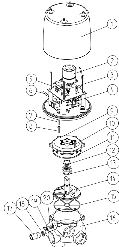
Рис. 9.3: Демонтаж вентиля
