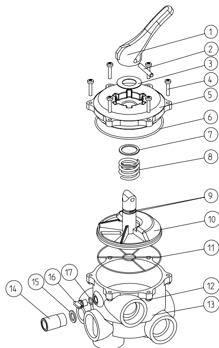
Рис. 9.3: многоходовой вентиль
