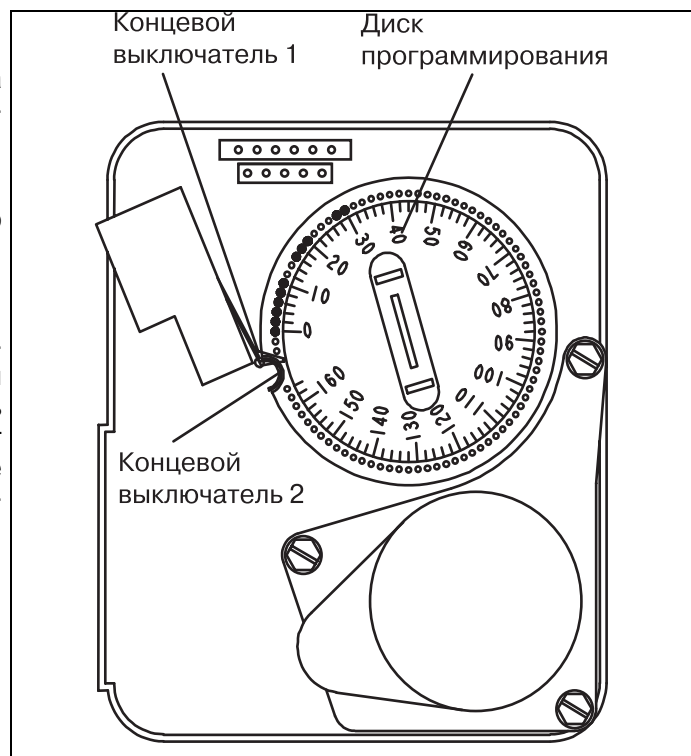
Рис. 11.2: Диск обратной промывки
