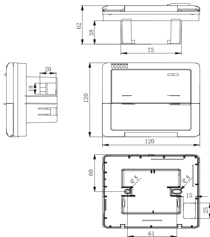
Рис. 6.20 Установочные размеры
