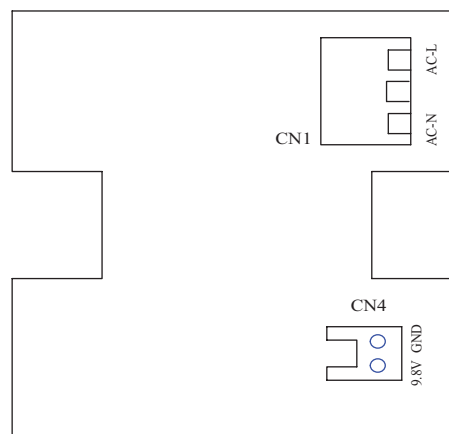
Рис. 6.22 Подключение электропитания
