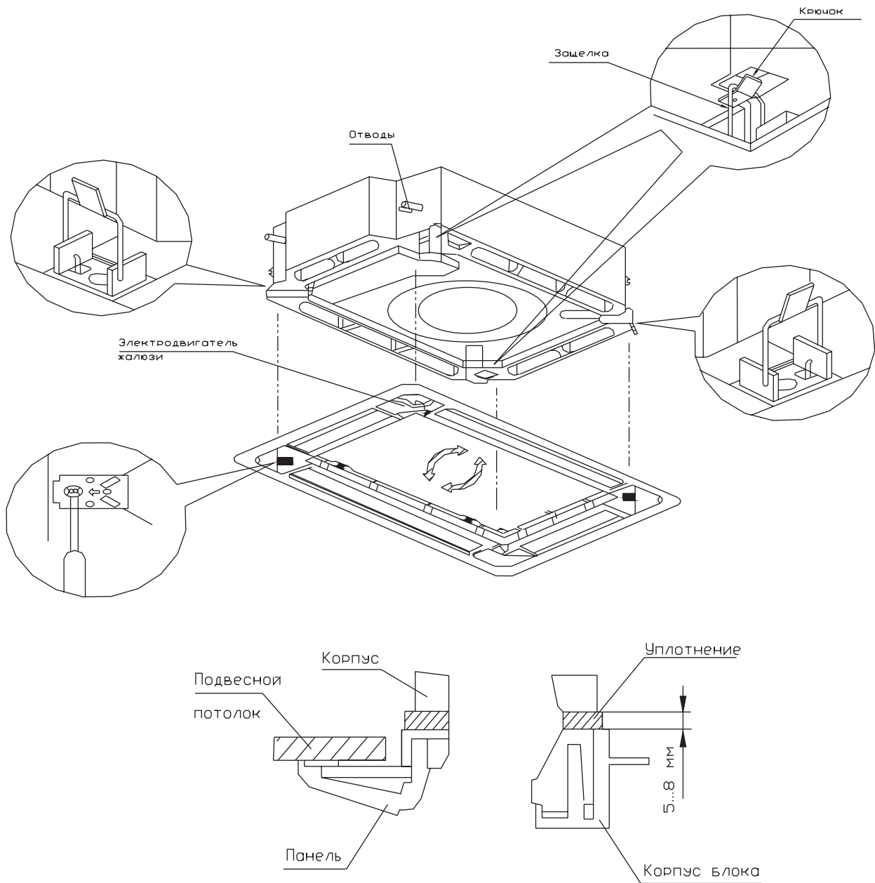
Рис. 10.20 — Установка панели
