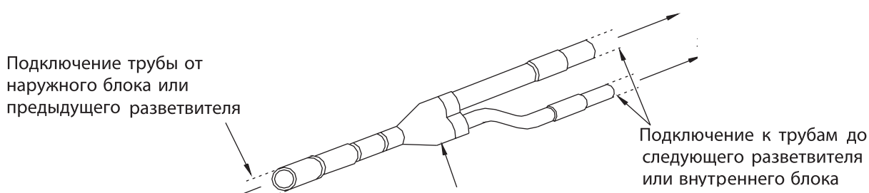
Рис. 11.4 — Подключение разветвителя
