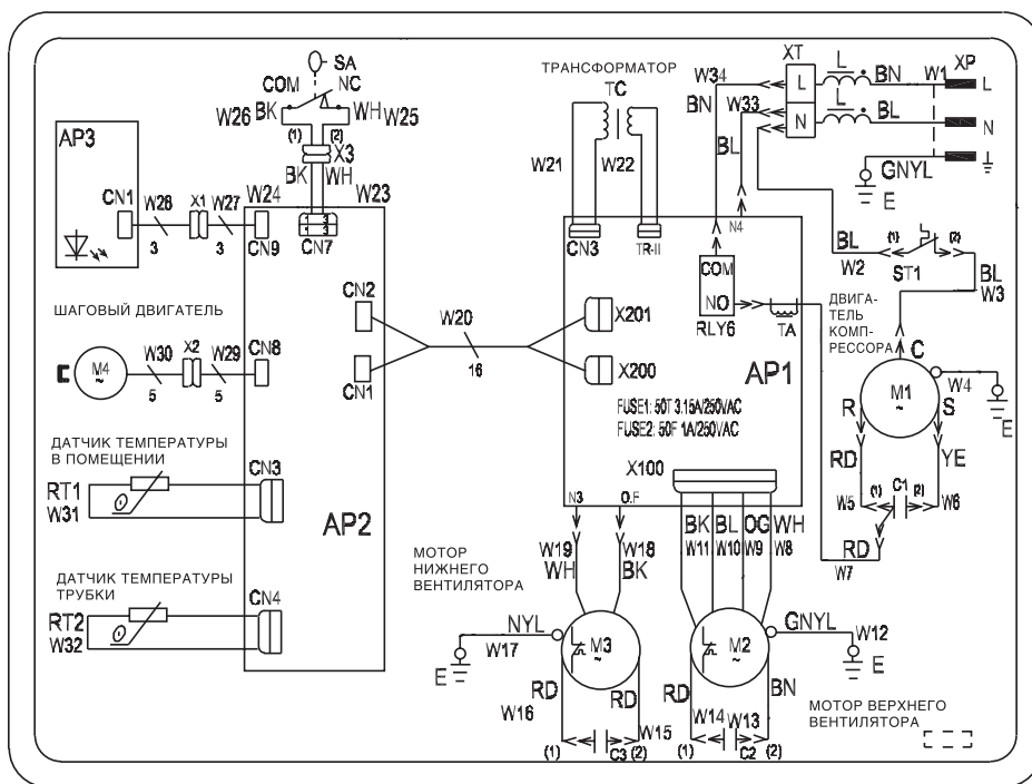
Схема электрическая функциональная
