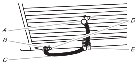
A. Пробка D. Зажим B. Отвод дренажный E. Фиксатор C. Трубка дренажная
