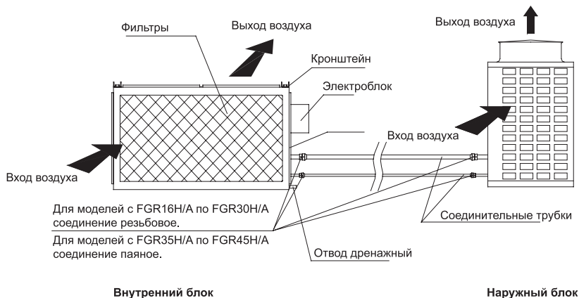
Рисунок 4.1 – Состав кондиционера
