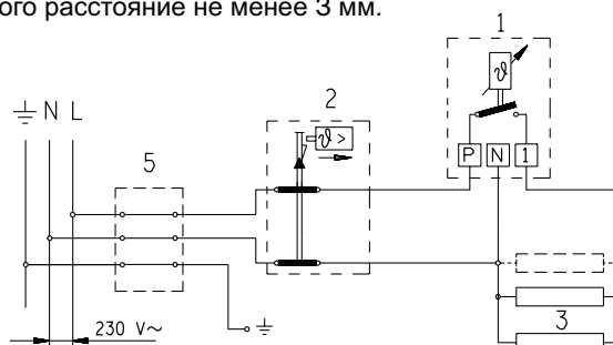
Электрическая схема
