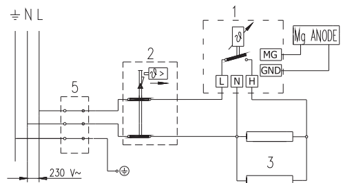
Elektroschema
