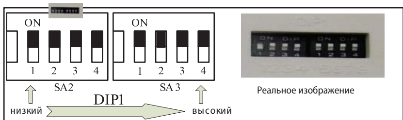
Рис. 6.43 Настройка DIP1
