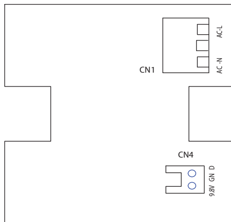
Рис. 6.22 Подключение электропитания
