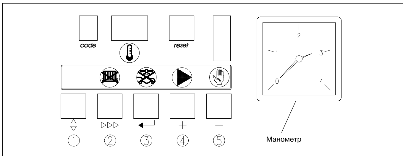
Abb.3: Панель управления
