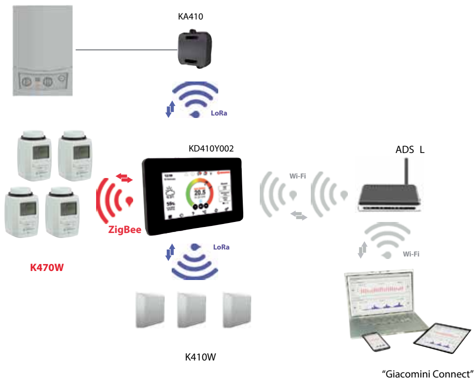
Схема работы системы управления отоплением "KLIMAdomotic" с терморегуляторами K470W
