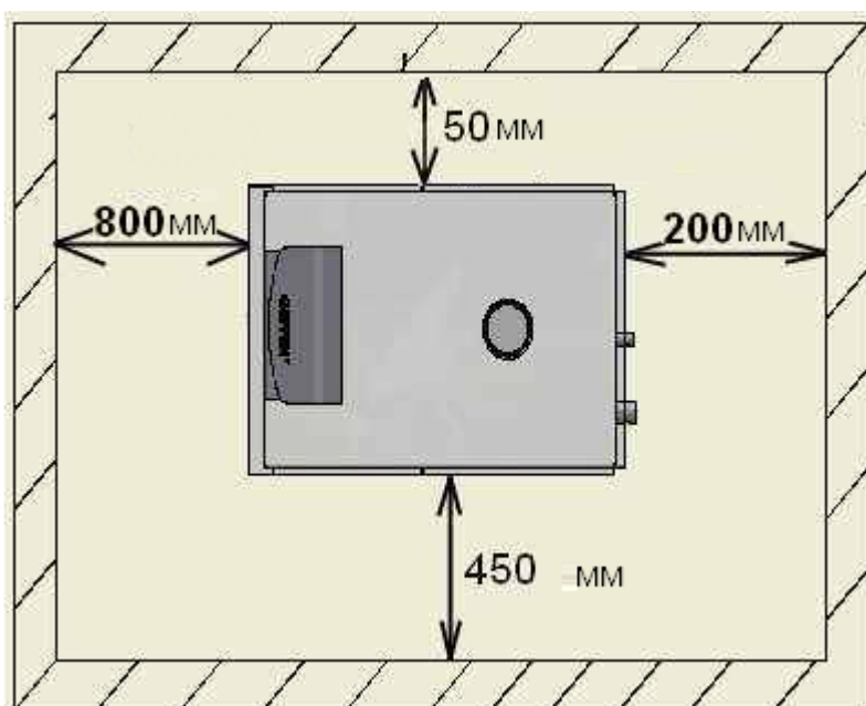
Котлы GEFLEN MB187, MB220, MB250, MB300
