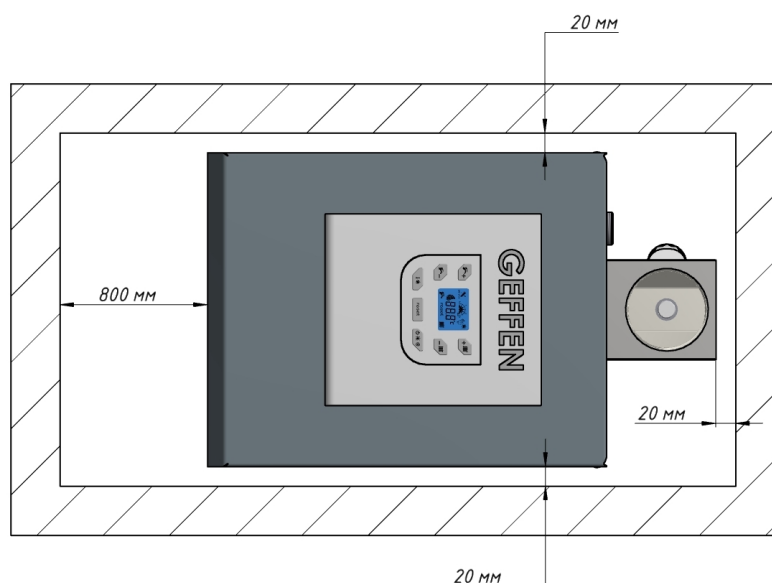
Рисунок 1. Монтаж котла GEFREN MB 4.1
