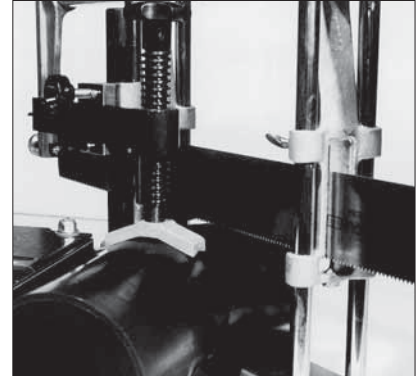
Обрезка фитинга
