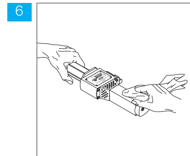
Очистить инструмент
