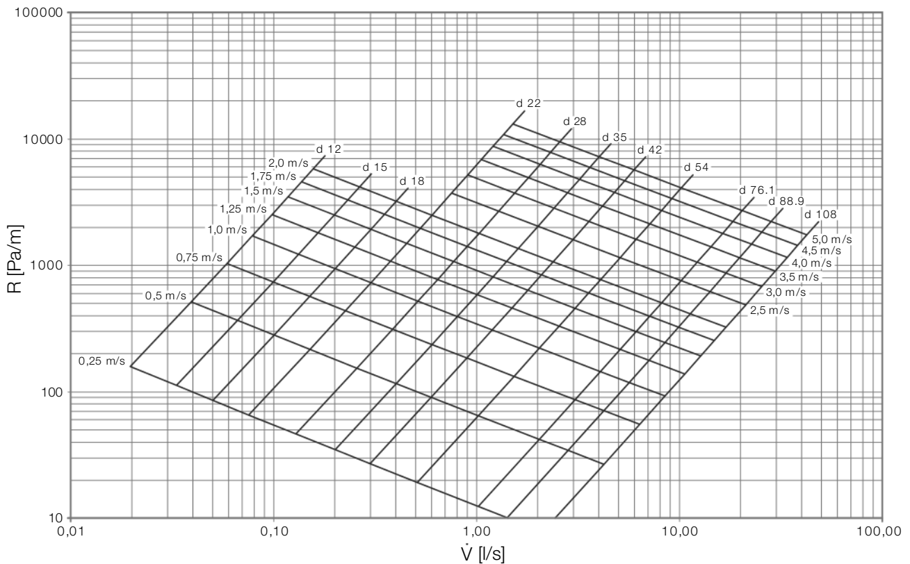
Рисунок 2: Потеря давления в трубопроводах из нержавеющей стали для теплой питьевой воды Geberit Mapress
