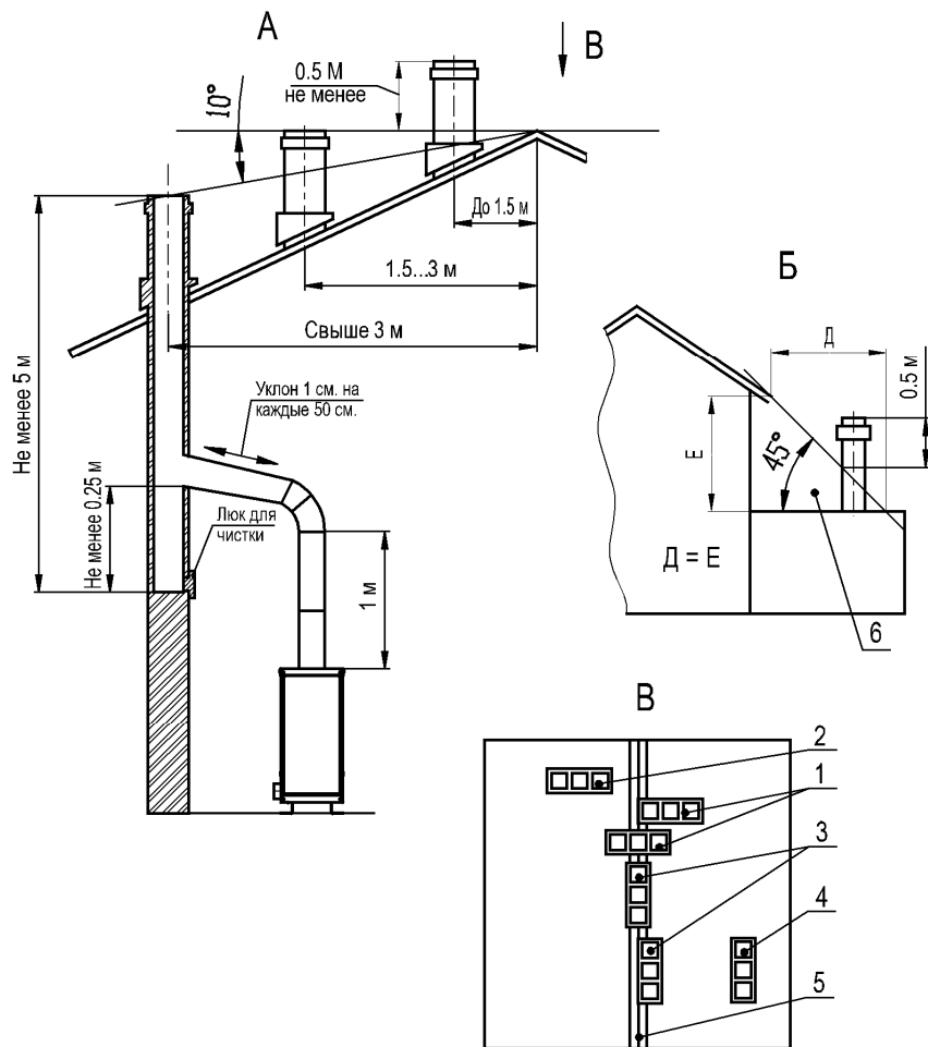
Рис.5 Схема расположения дымовой трубы и котла
