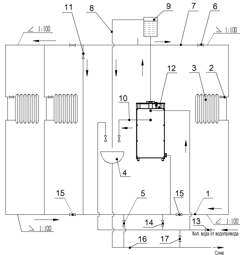
Рис.6 Рекомендуемая схема системы отопления котла
