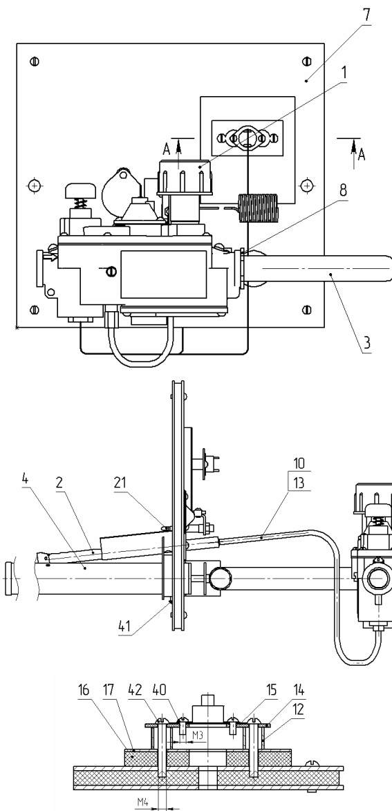
1-блок управления; 2-блок запальника; 3-коллектор; 4-труба горелочная; 7-панель; 8-гайка; 10-трубка запальника; 12-штулка; 13-прокладка; 14-панель; 15-шайба; 16-теплоизоляция; 17-пластина; 21-термопара; 40-винт М3; 41-винт М4х8; 42-винт М4х22
