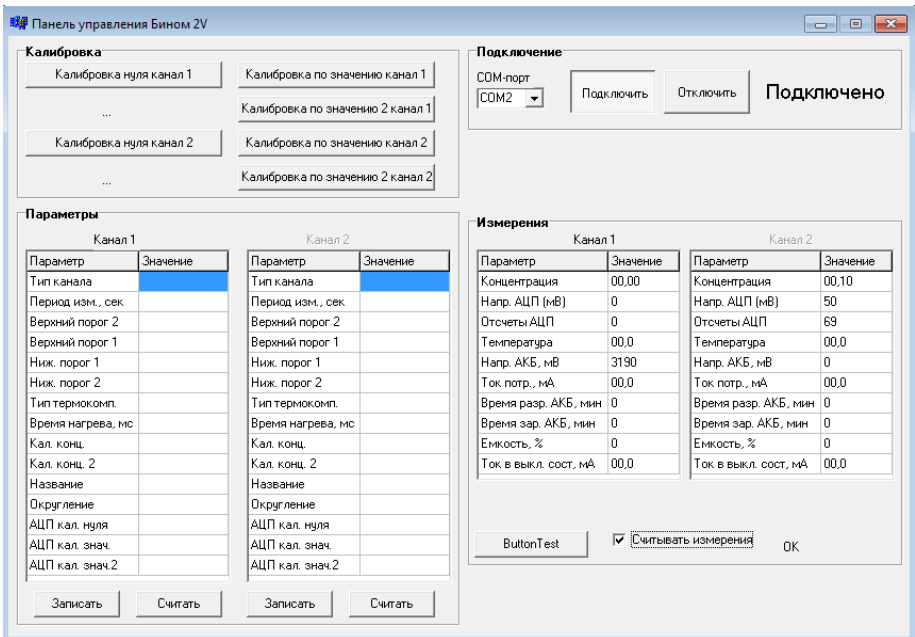
Рисунок 4. Установка соединения
