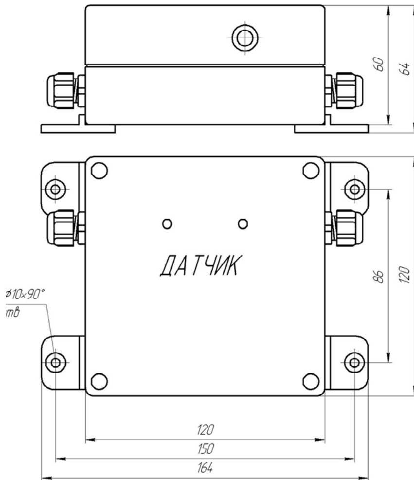
Рис 6. Габариты датчика
