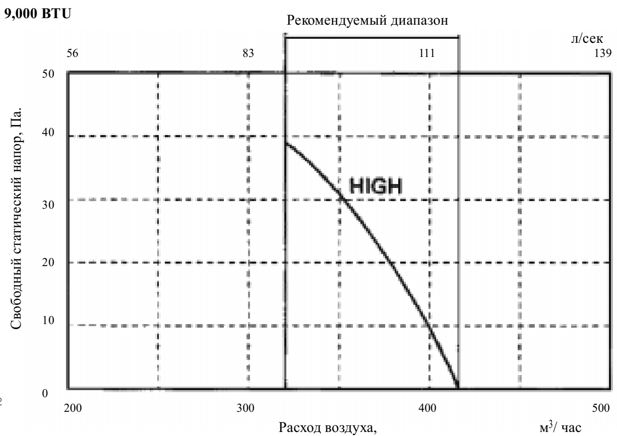
Рис. 48 Зависимость расхода воздуха и свободного статического напора вентилятора
