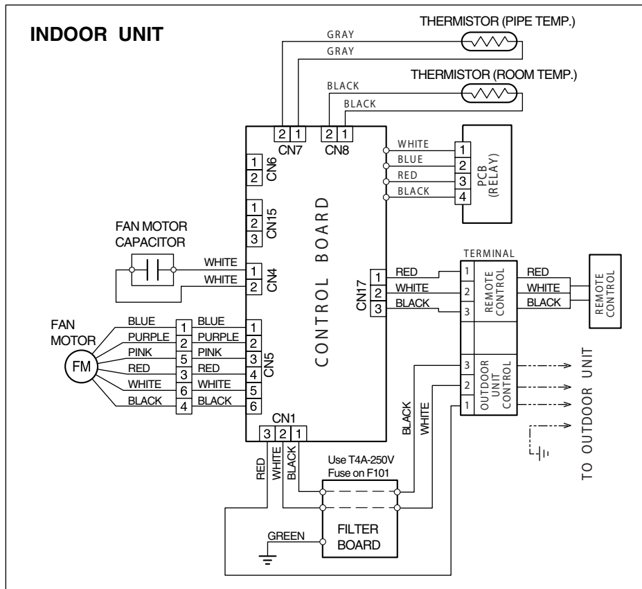
FAN MOTOR CAPACITOR 10.0 μF
