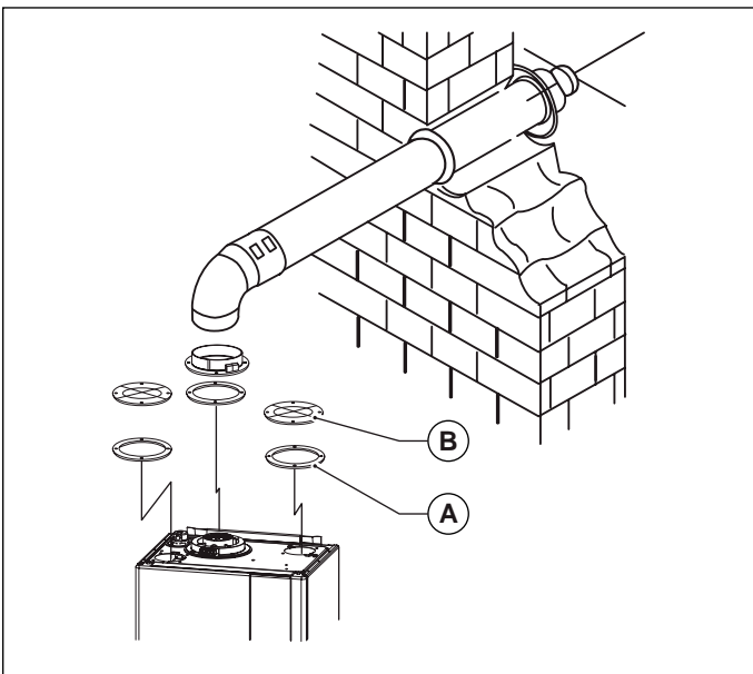
Рис. 11 Коаксиальная система воздухозабора и дымоотвода типа С33
