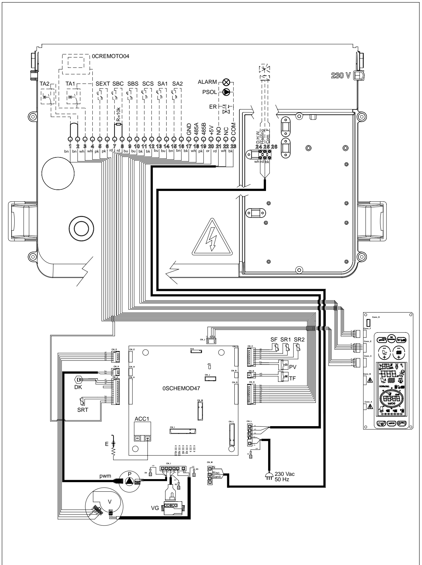
Рис. 29 Электрическая схема KR
