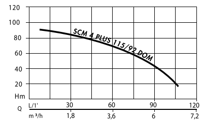
Кривая производительности
