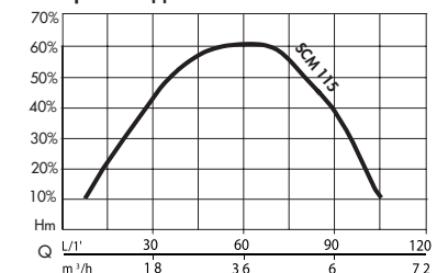
Кривая производительности
