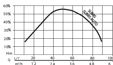
Кривая производительности
