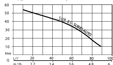
Кривая производительности
