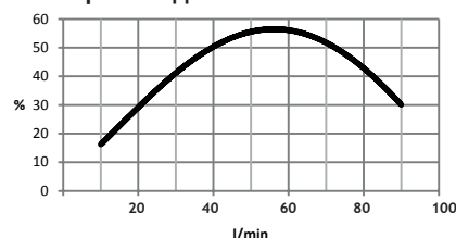
Кривая производительности
