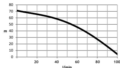
Кривая производительности
