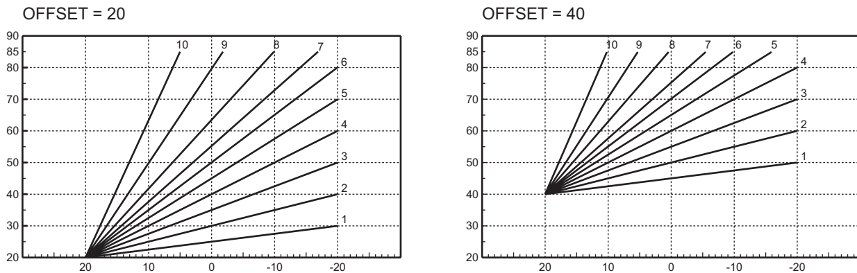
рис. 13 - Пример параллельного смещения компенсационных характеристик
