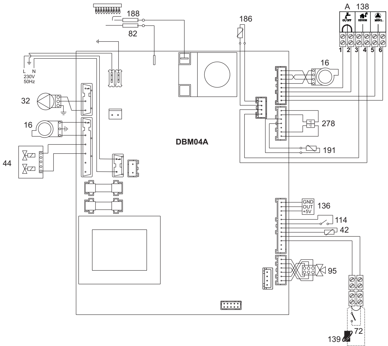
рис. 33 - Электрическая схема
