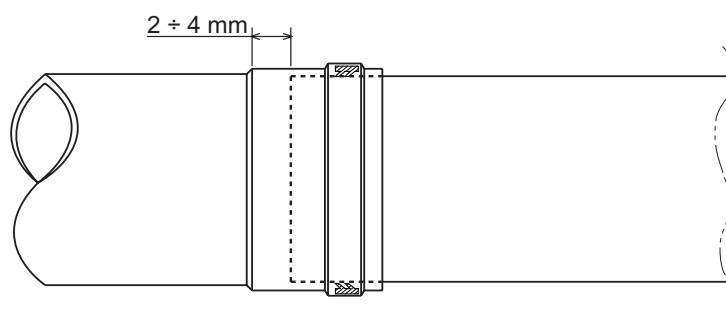
рис. 19 - Тепловое расширение
