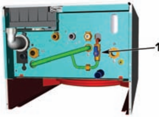
рис. 15 - Кран для заполнения системы отопления
