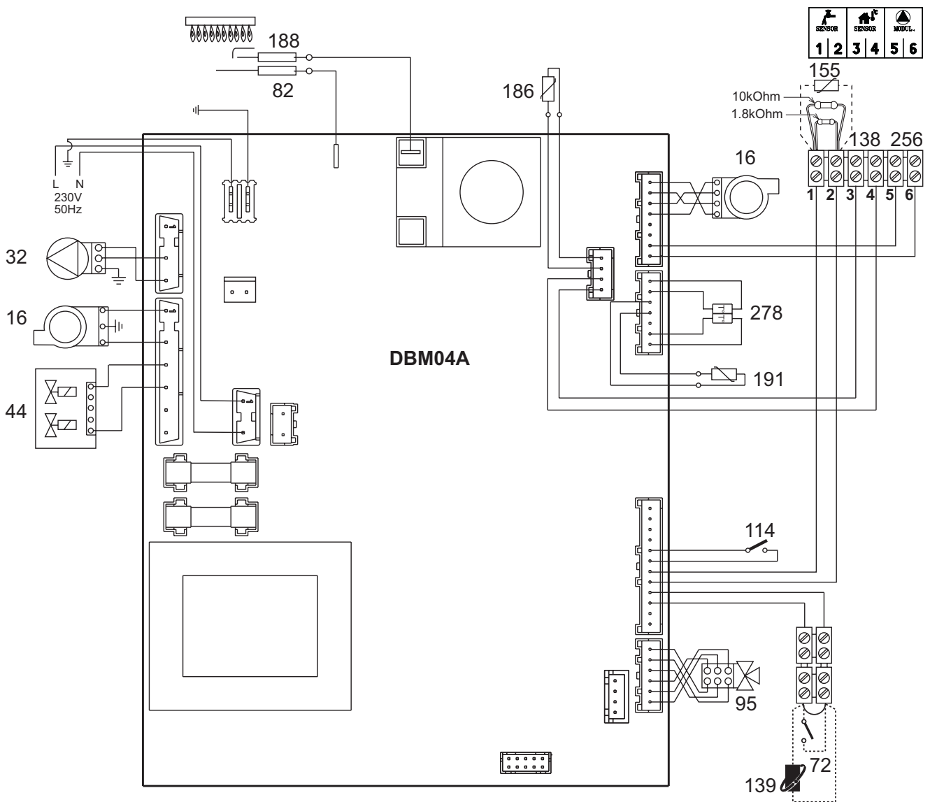
рис. 34 - Электрическая схема
