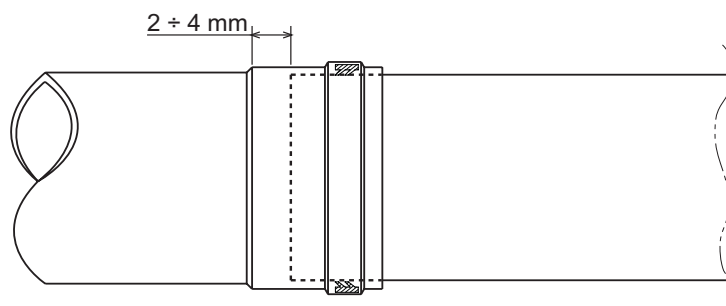
рис. 20 - Тепловое расширение
