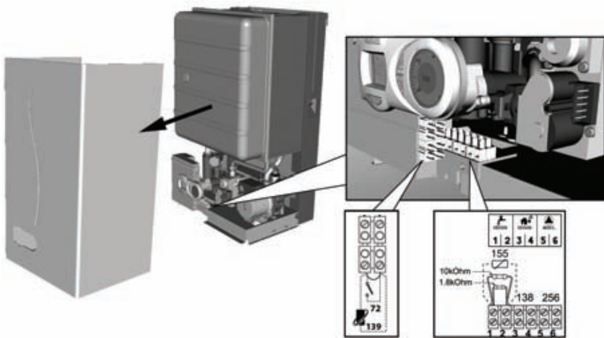
рис. 19 - Доступ к блоку зажимов
