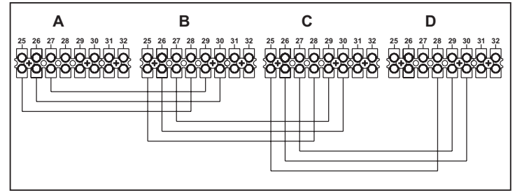
мал. 23 - Каскадне підключення
