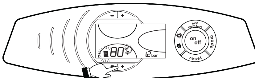
рис. 15 - Работа в режиме TEST
