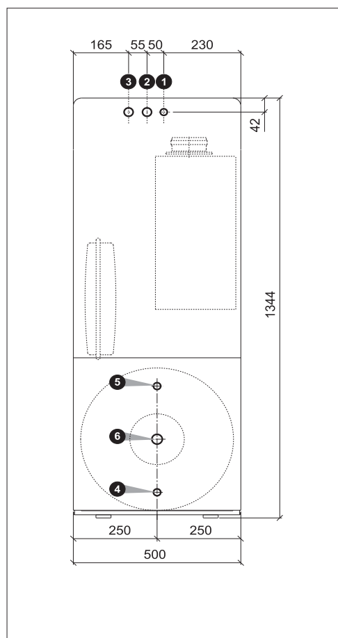
Рис. 3 Вид сзади
