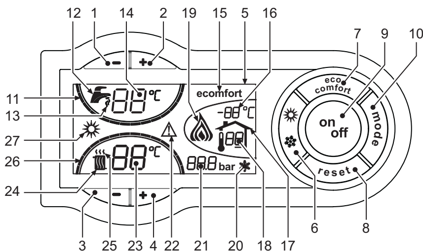
рис. 1 - Панель управления
