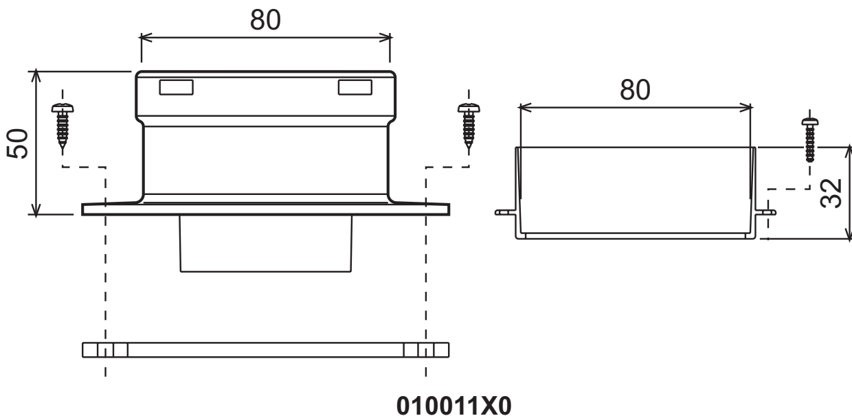
рис. 24 - Соединительный элемент для отдельных труб
