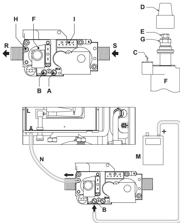
рис. 27 - Газовый клапан
