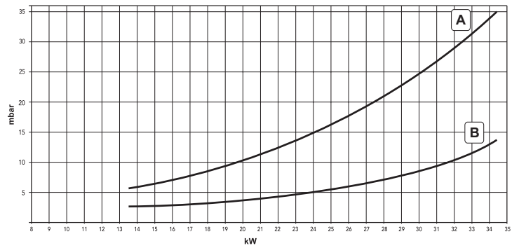
fig. 35 - Diagrama presión / potencia DIVAtop MICRO F 32
