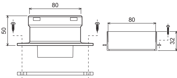
рис. 24 - Соединительный элемент для отдельных труб
