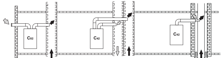
fig. 25 - Ejemplos de conexión a chimeneas (⇨ = aire / ⇩ = humos)
