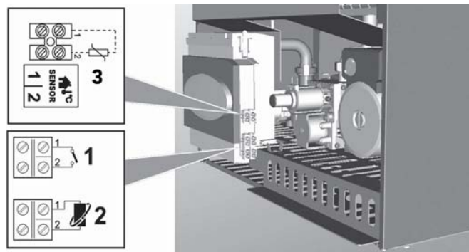
рис. 20 - Доступ к клеммной коробке
