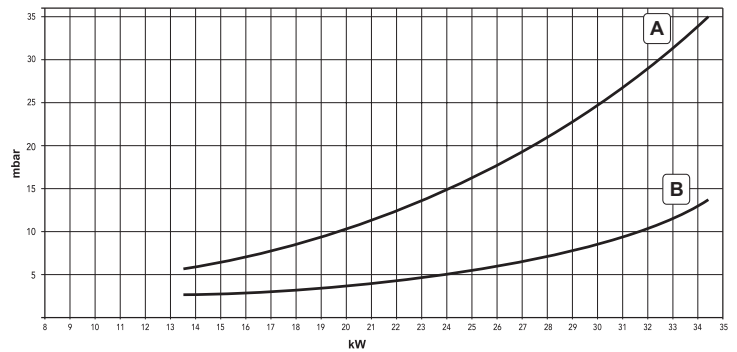
fig. 35 - Diagramă presiune/putere DIVAtop MICRO F 32
