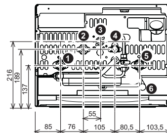
fig. 17 - Racordurile hidraulice
