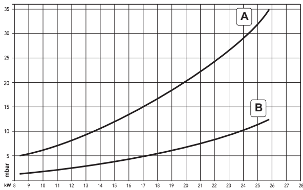
fig. 33 - Diagrammes pression - puissance DIVAtop MICRO F 24
