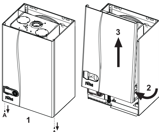
fig. 28 - Deschiderea carcasei
