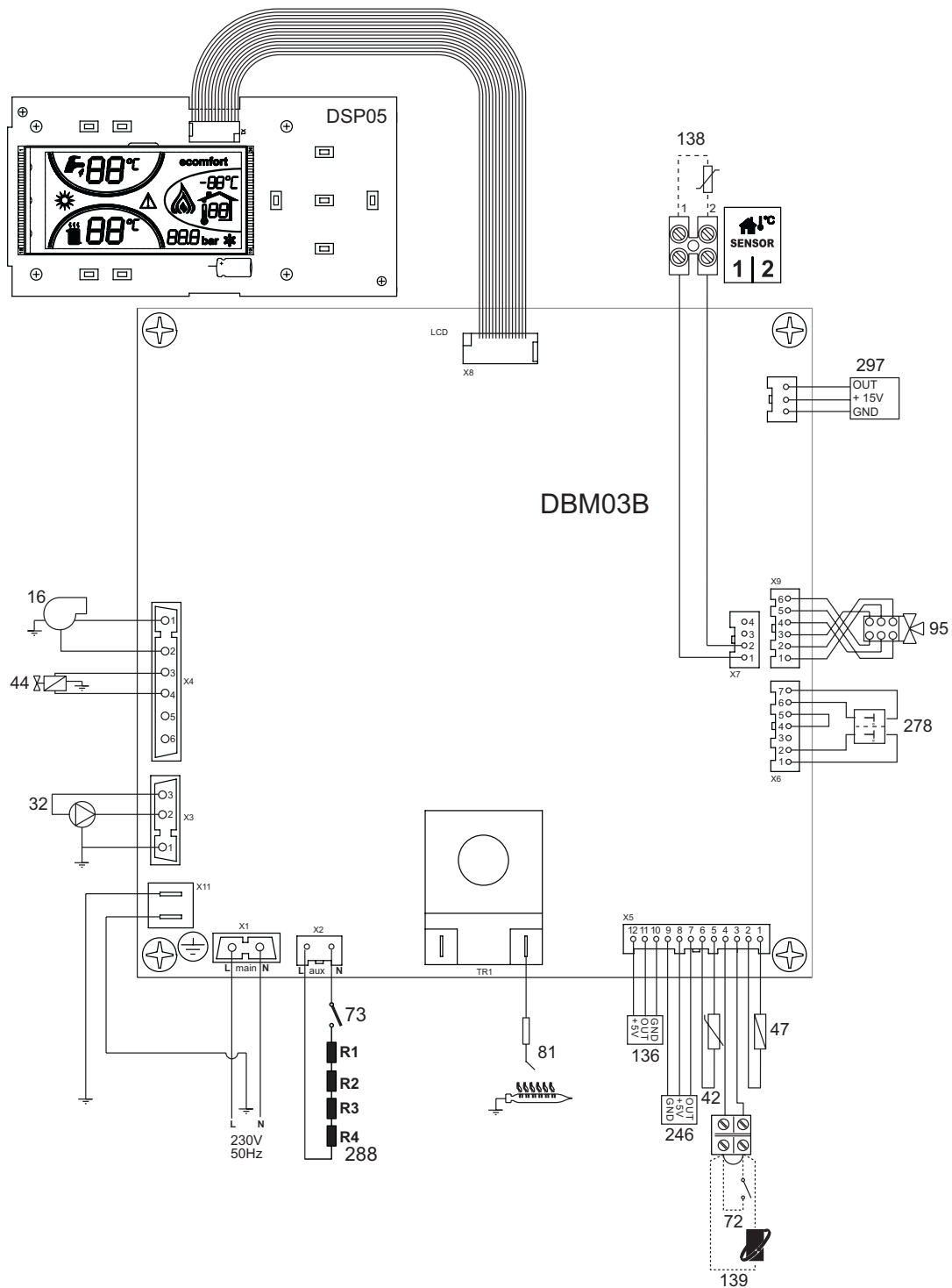
fig. 39 - Schema elettrico
