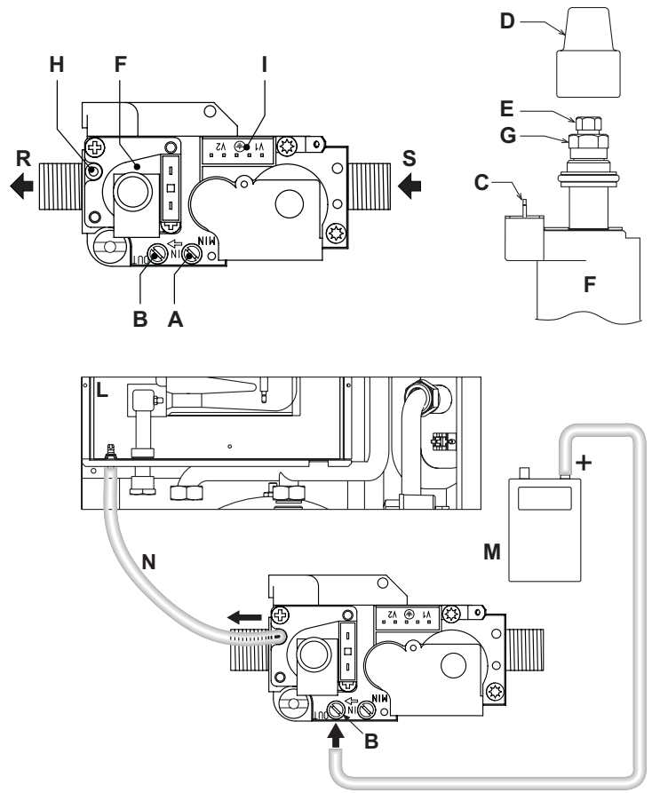
şek. 27 - Gaz valfi
