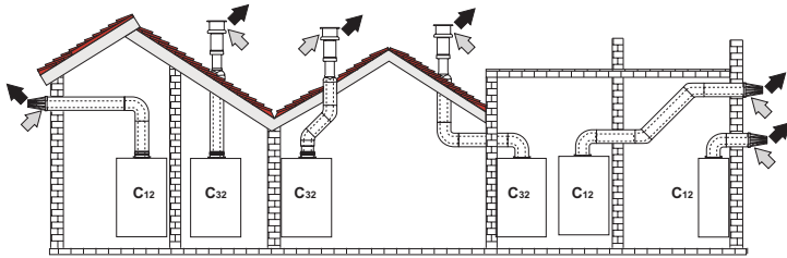
мал. 21 - Приклад підключення за допомогою співісних (коаксiальних) труб (⇨ = Повітря / ⇨ = Відпрацьовані гази)
