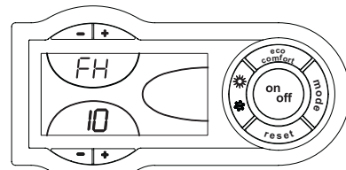
fig. 6 - Aprinderea centralei
