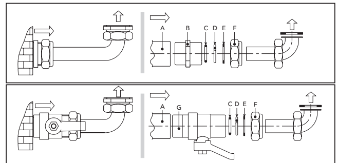
рис. 18 - Соединительный комплект
