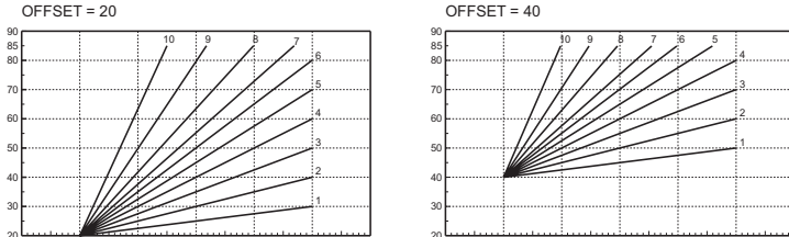
мал. 15 - Пříklad паралельного пересування компенсаційних кривих
