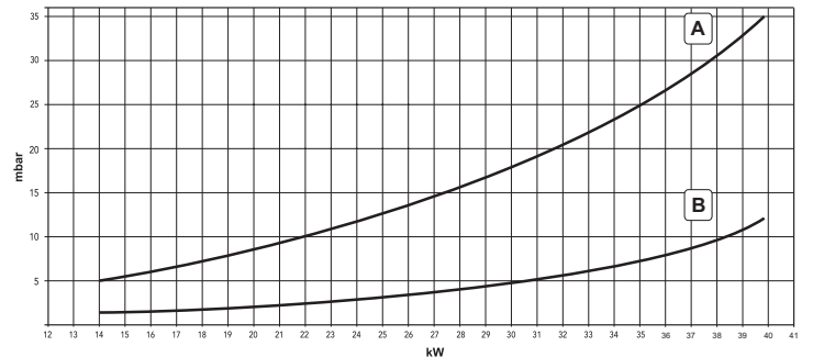
fig. 37 - Diagrammes pression/puissance DIVAtop MICRO F 37
