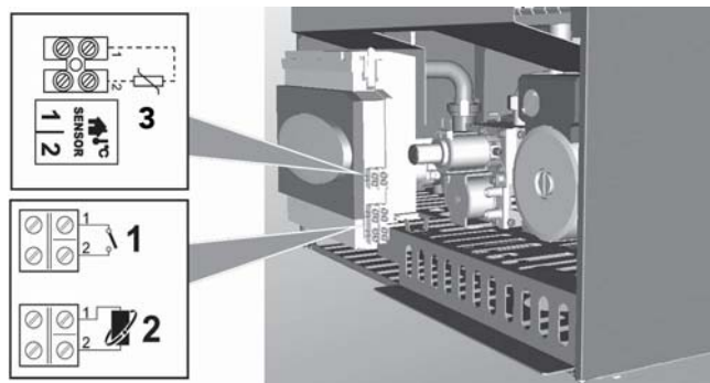
мал. 20 - Доступ до клемної коробки
