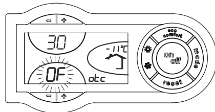
fig. 13 - Deplasarea paralelă a curbelor
