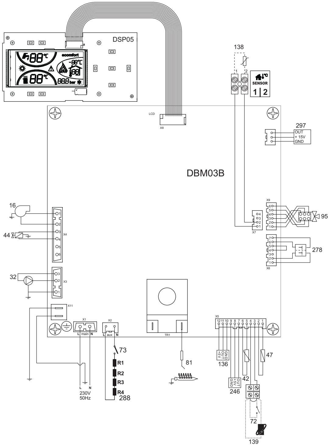
fig. 39 - Esquema eléctrico
