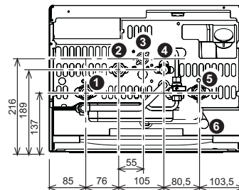
fig. 17 - Conexiones hidráulicas
