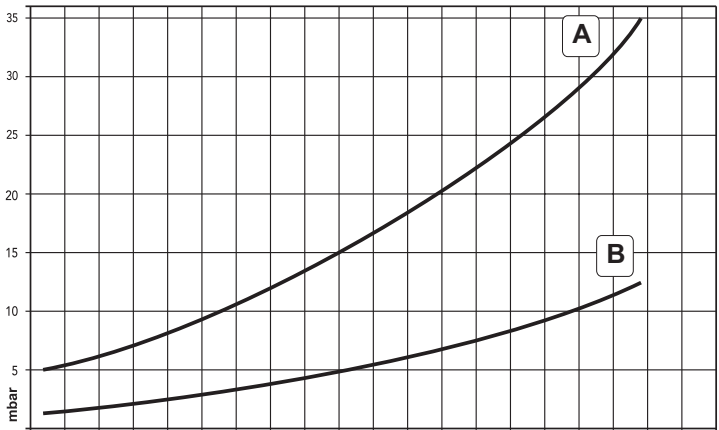
мал. 33 - Діафрагма тиску/потужність DIVAtop MICRO F 24
