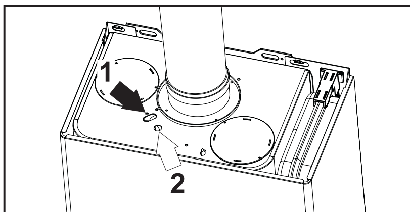
рис. 18 - Анализ продуктов сгорания
