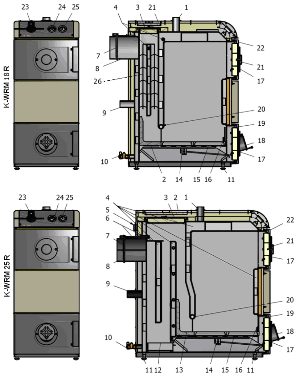
Рисунок 1. Схема строения котла.
