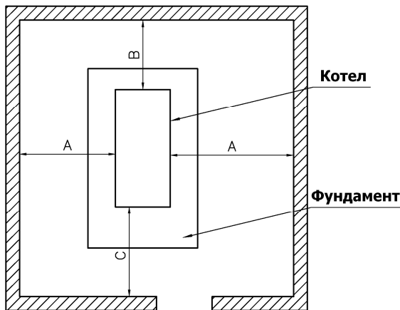
Рисунок 3 Расстояния между котлом и стенами
