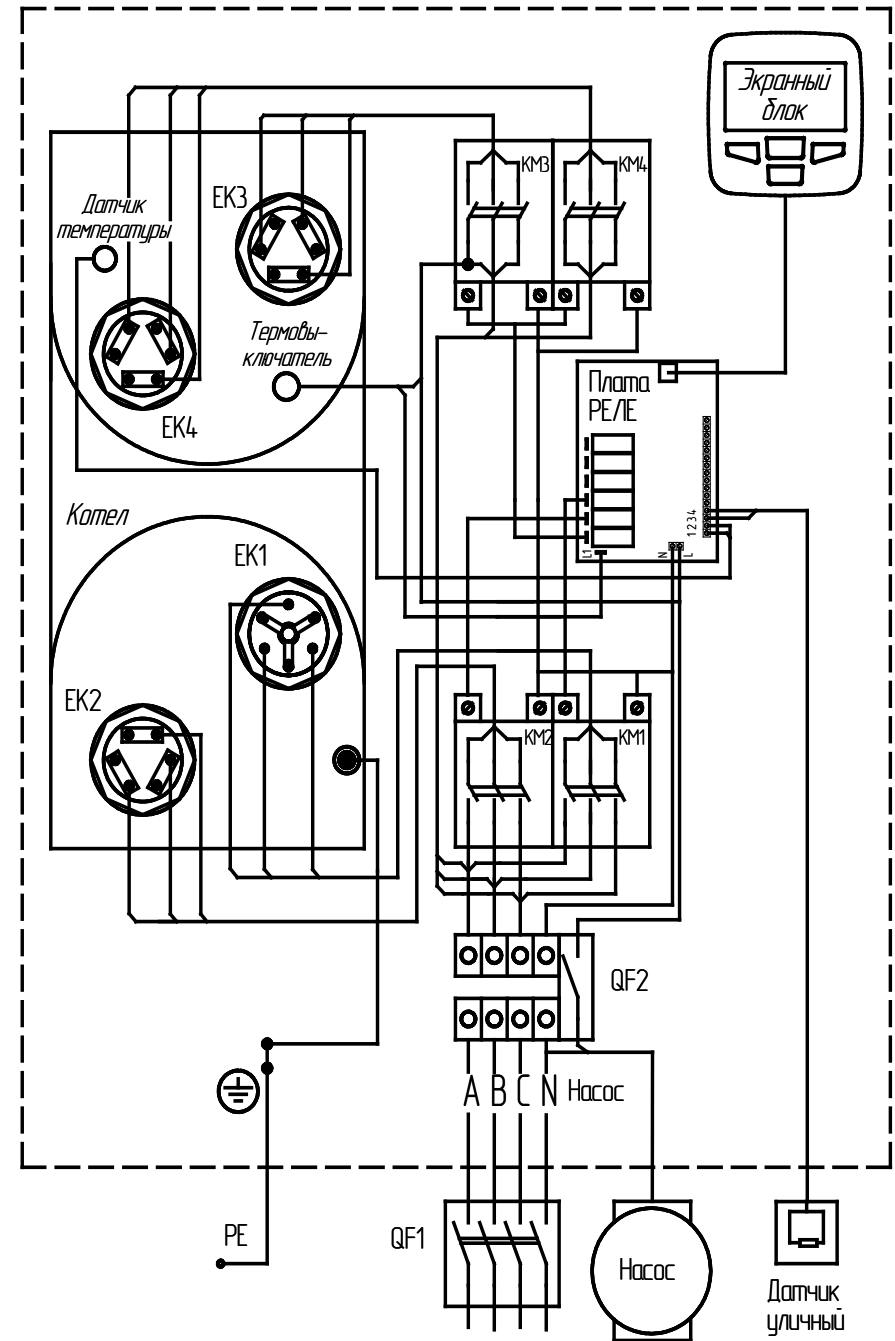
Рисунок 7. Схема подключения ЗВАН UNIVERSAL -4,8, 54 - 13 -
